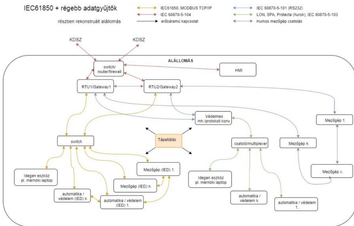
15.2. ábra: Részben felújított adatgyűjtő rendszer
