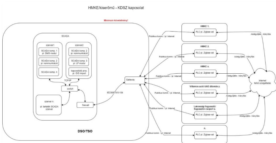
15.9. ábra: HMKE-Aggregátor-SCADA kapcsolat
