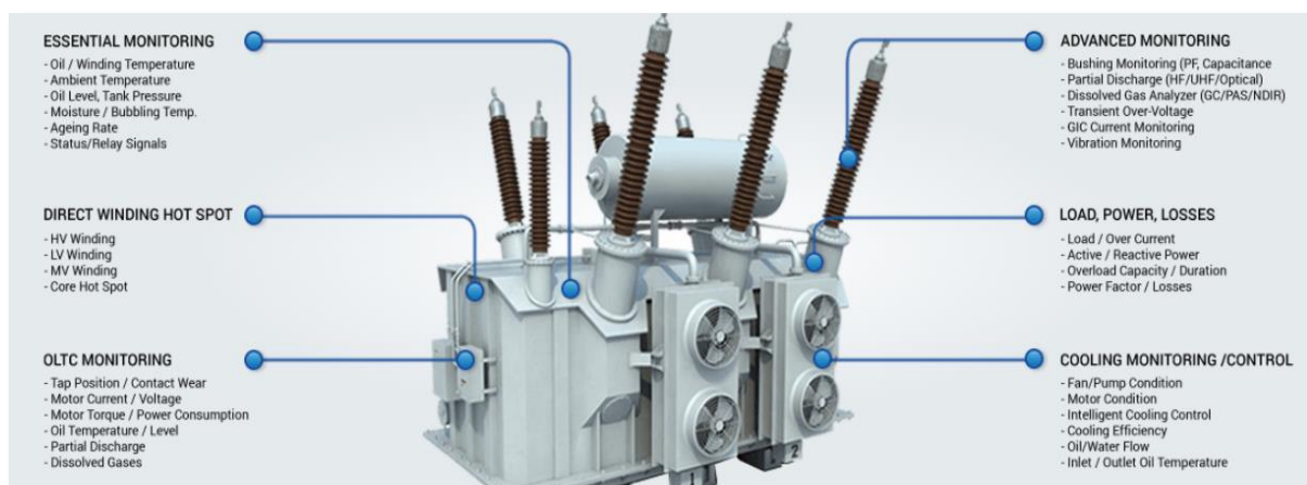
7.2. ábra: Nagytranszformátor Purdue 0. és 1. szintű eszközei, berendezése 217
