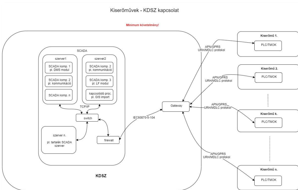
15.10. ábra: Kiserőmű-KDSZ
