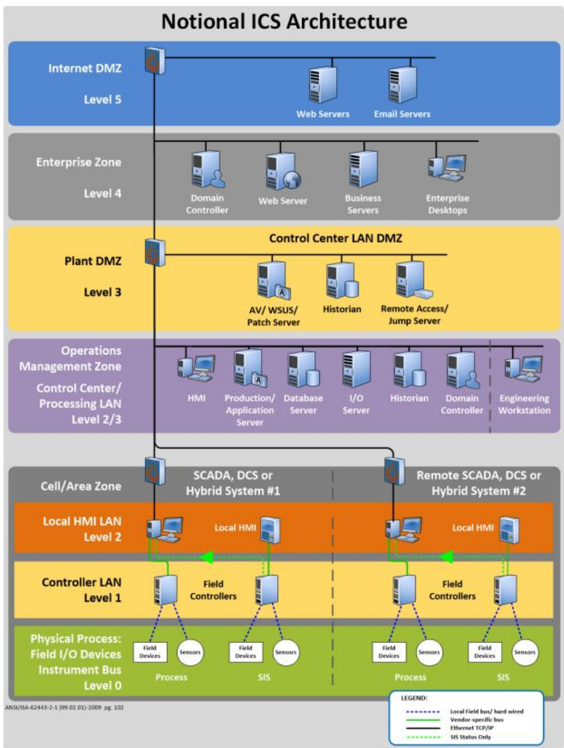
9. ábra: A Purdue modell az OSTI 107 ábrázolásában 108 [8]
